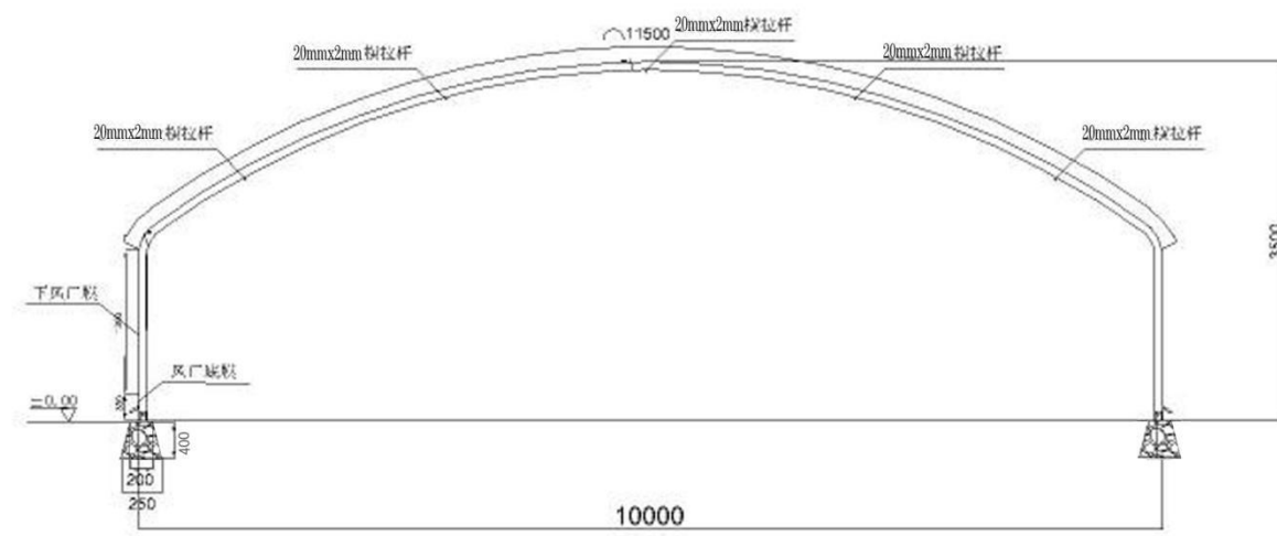
10米跨拱棚剖面图
