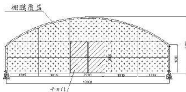
10米跨拱棚棚头立面图1
