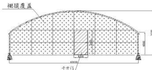
10米跨拱棚棚头立面图2
