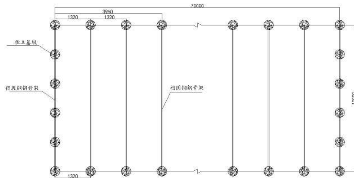
10米跨拱棚平面图
